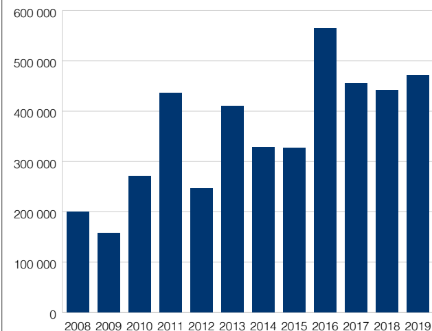
Figur 2.6: Vannskader på bygg som følge av vanninntrenging utenfra ved avrenning på bakken (ytte påvirkning) 2008 – 2019. Erstatningsbeløp i mill. kroner. Kilde: VASK, Finans Norge.
